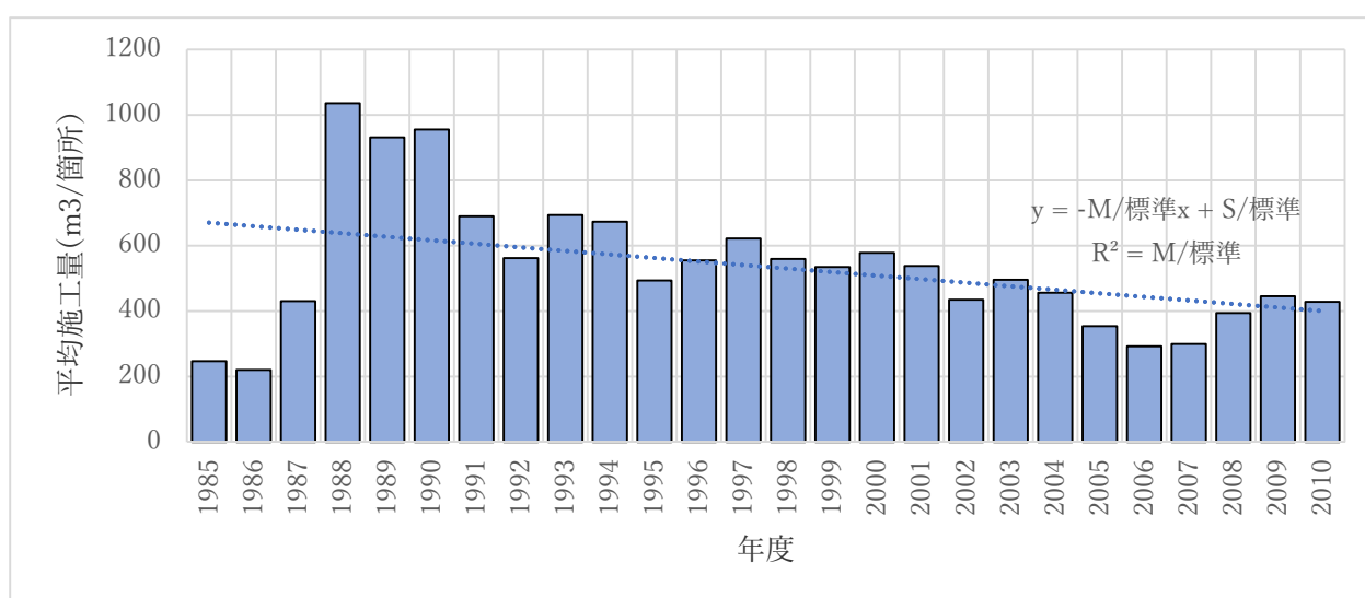
図-2 1現場当りの平均施工量の年別推移
