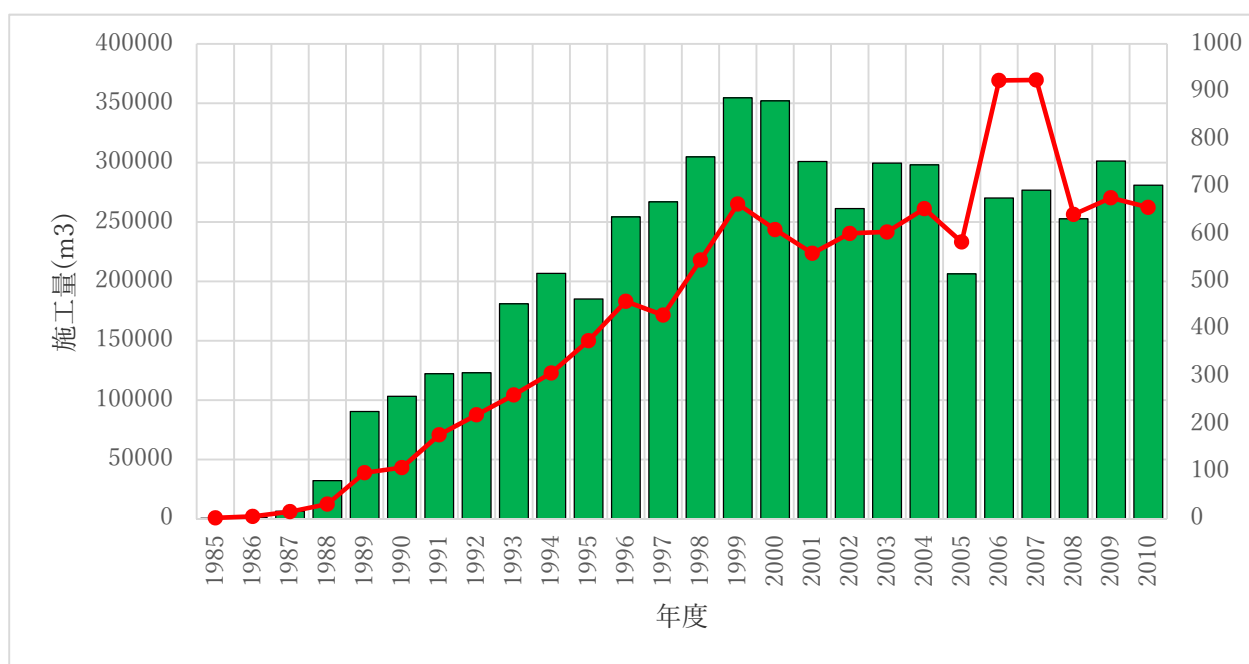
図-1 EPS全国実績の年別推移
