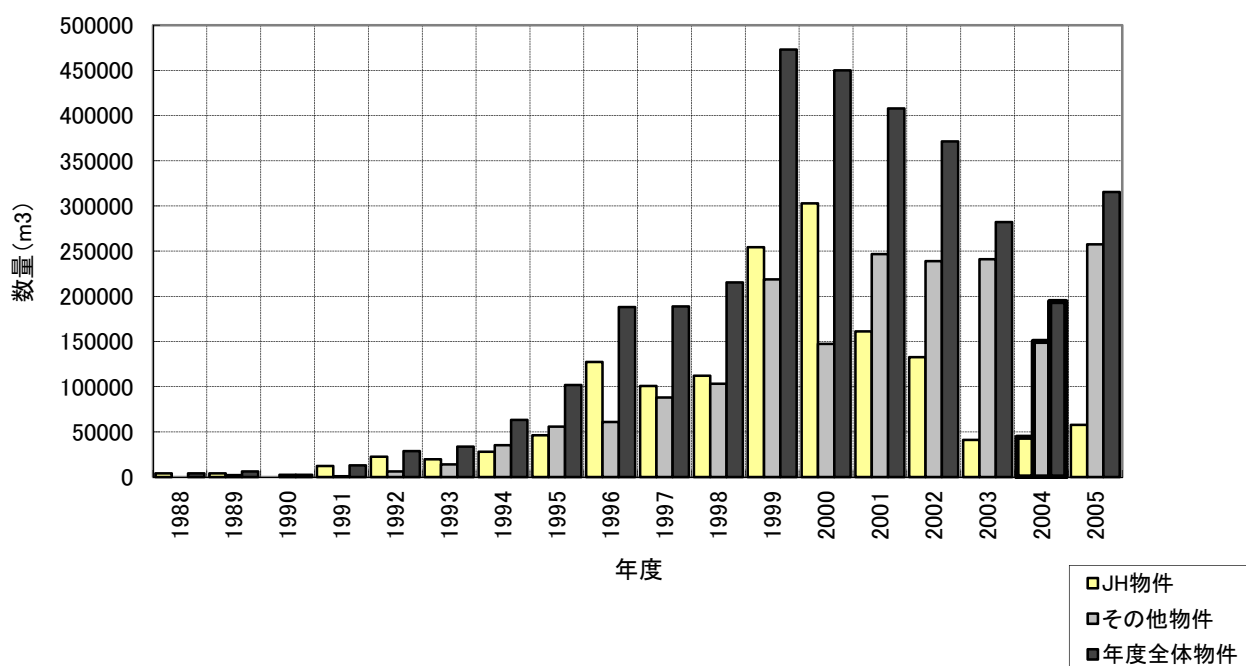
図-1 気泡混合軽量土の全国実績の年別推移
